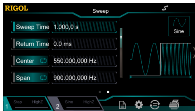
Figure 2-10 ステップ・スイープ
