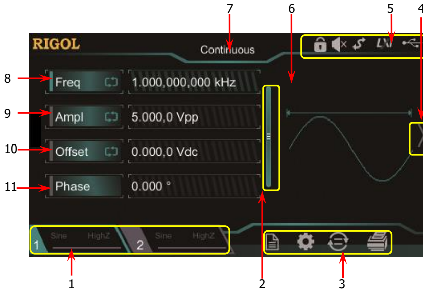
Figure 1-1 ユーザー・インタフェース
