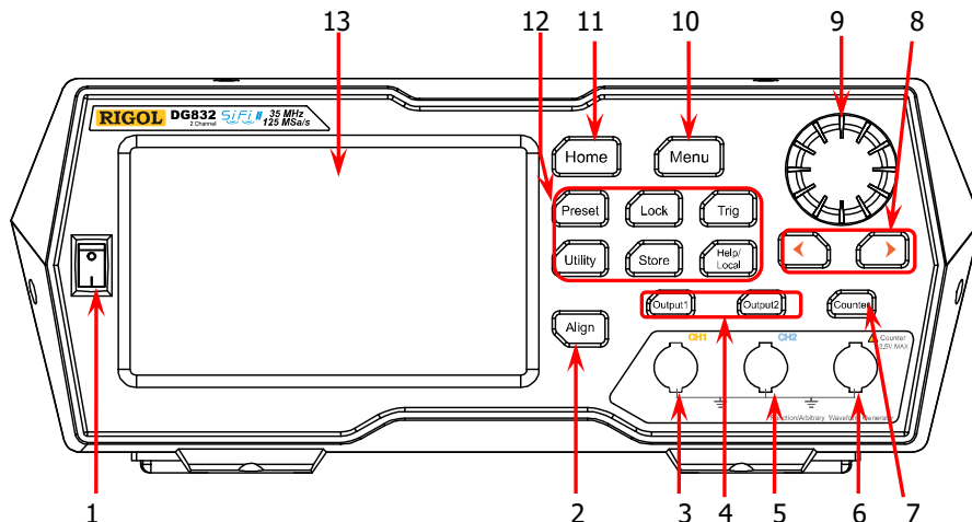
Figure 1-1 フロント・パネル
