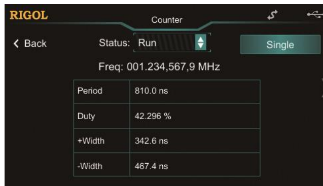
Figure 2-17 周波数カウンタ測定インターフェイス
