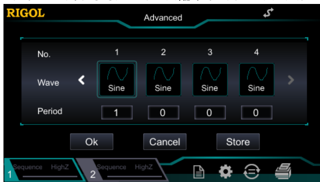
Figure 2-7 シーケンス編集インタフェース
